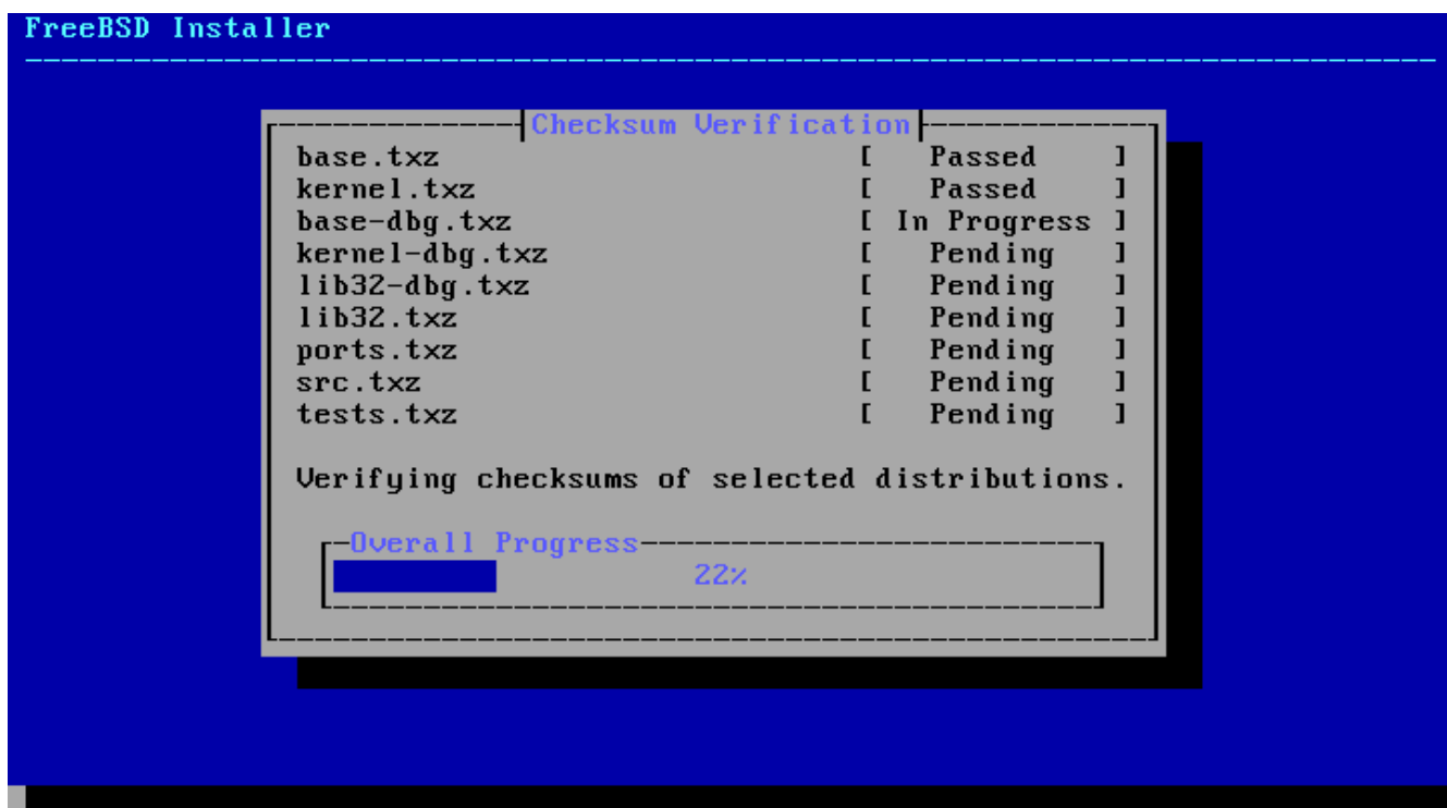
図 32. 配布ファイルの検証
