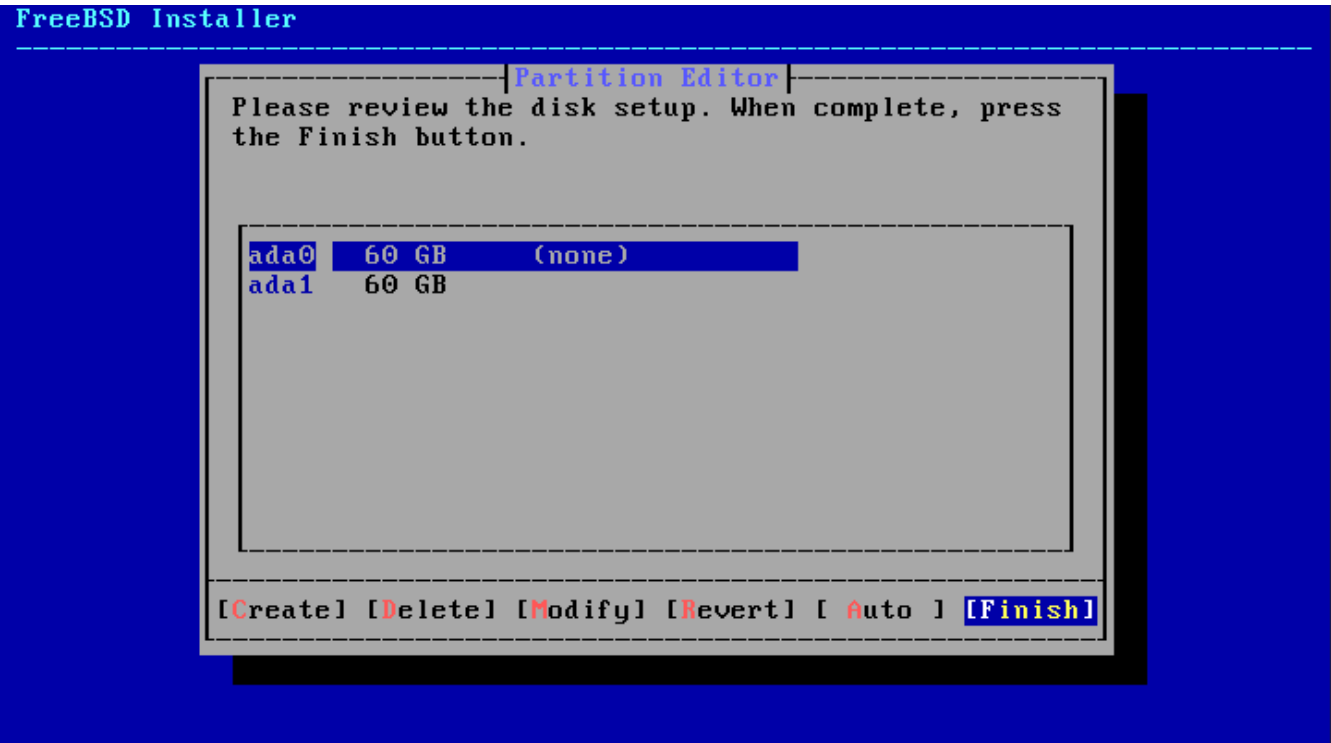
図 17. Manual によるパーティションの分割
