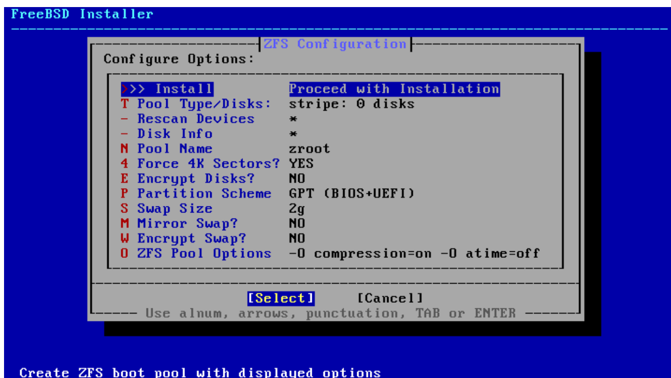
図 20. ZFS パーティションメニュー
