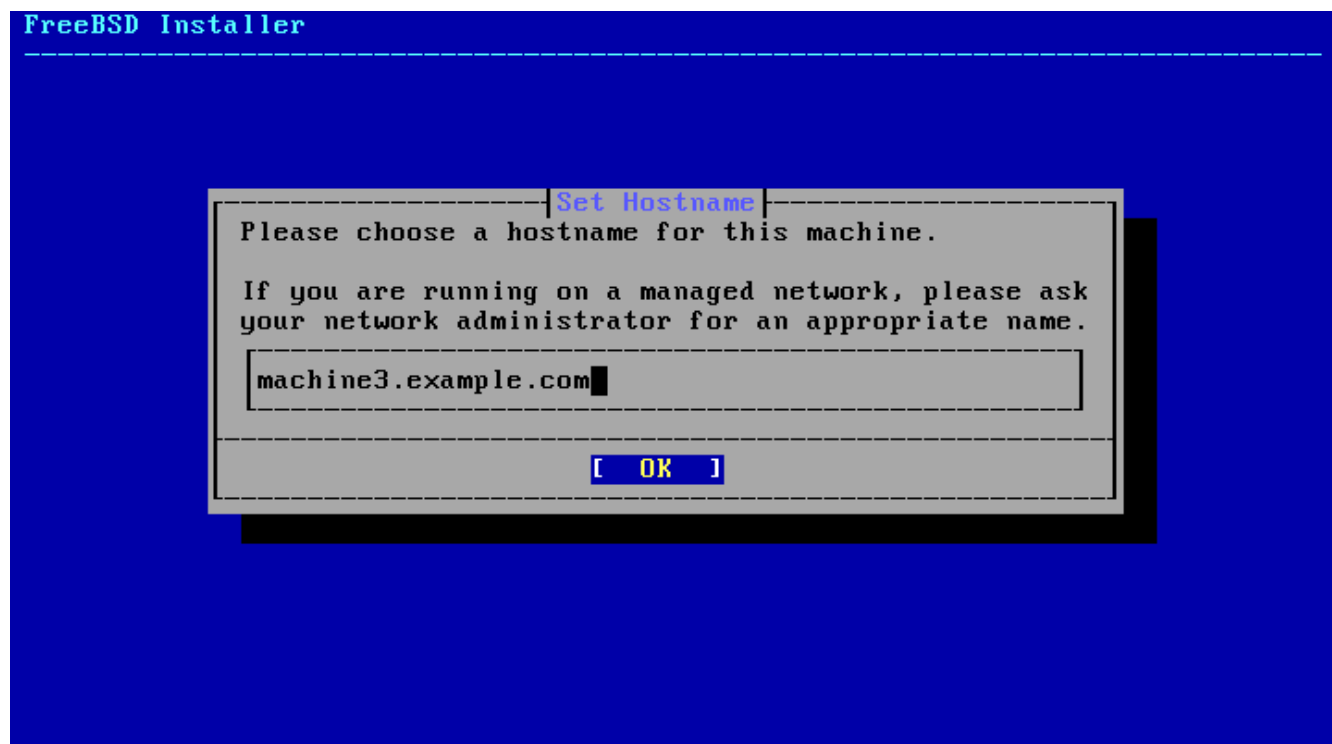
図 7. ホスト名の設定
