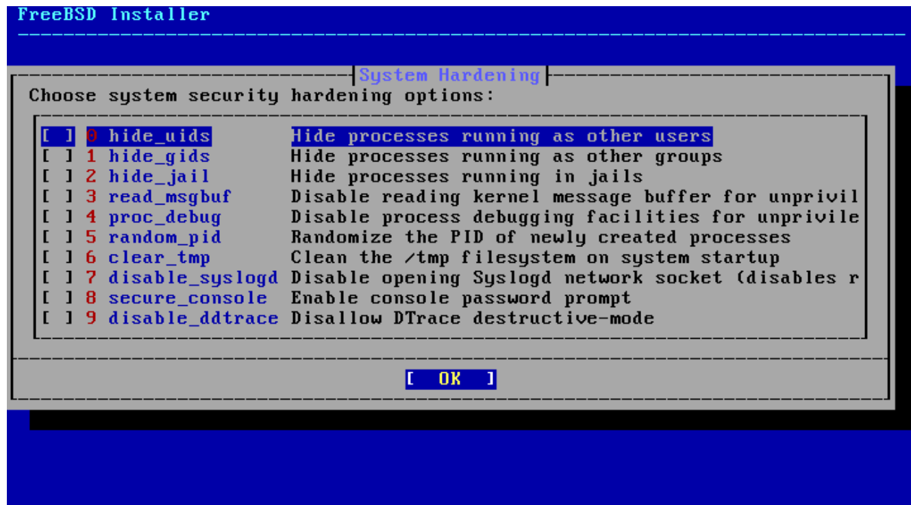
図 54. セキュリティを強化するオプションの設定
