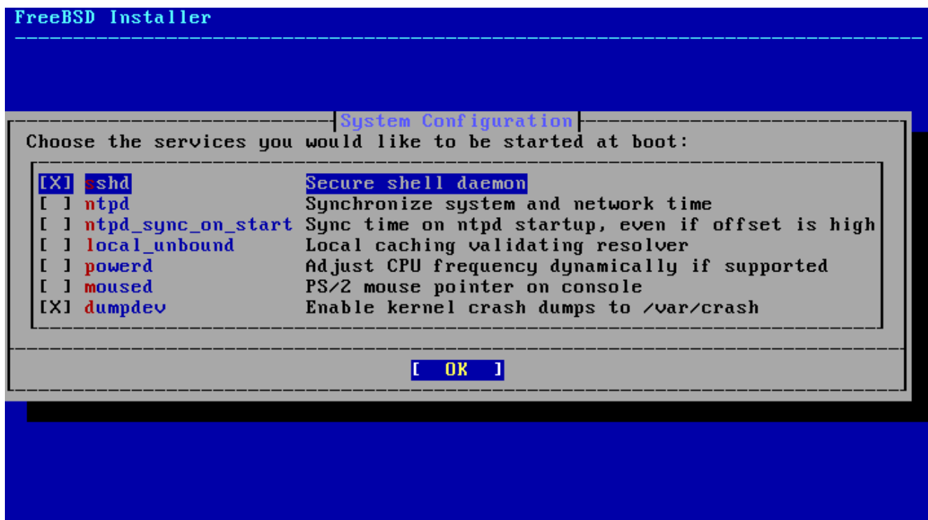
図 53. 追加で有効にするサービスの選択
