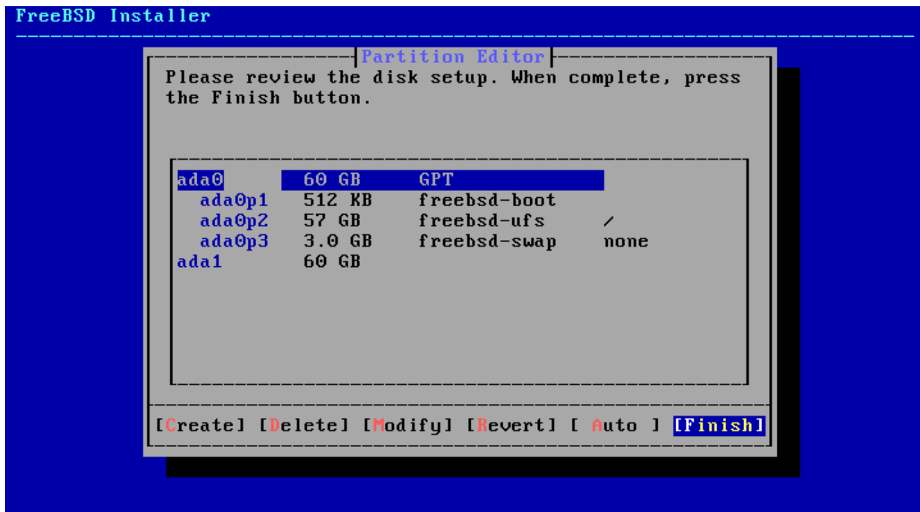
図 15. 作成されたパーティションの確認
