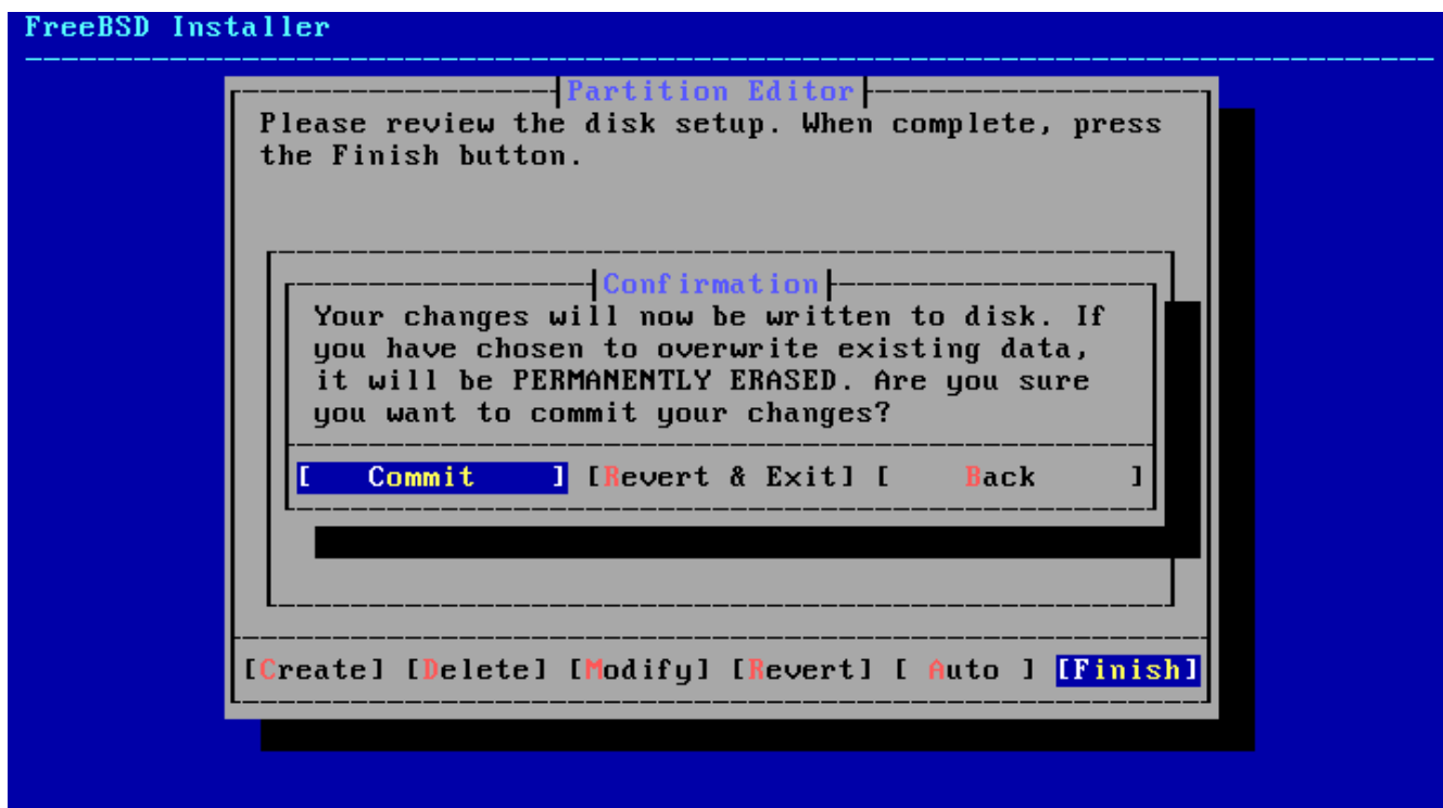
図 16. 最後の確認
