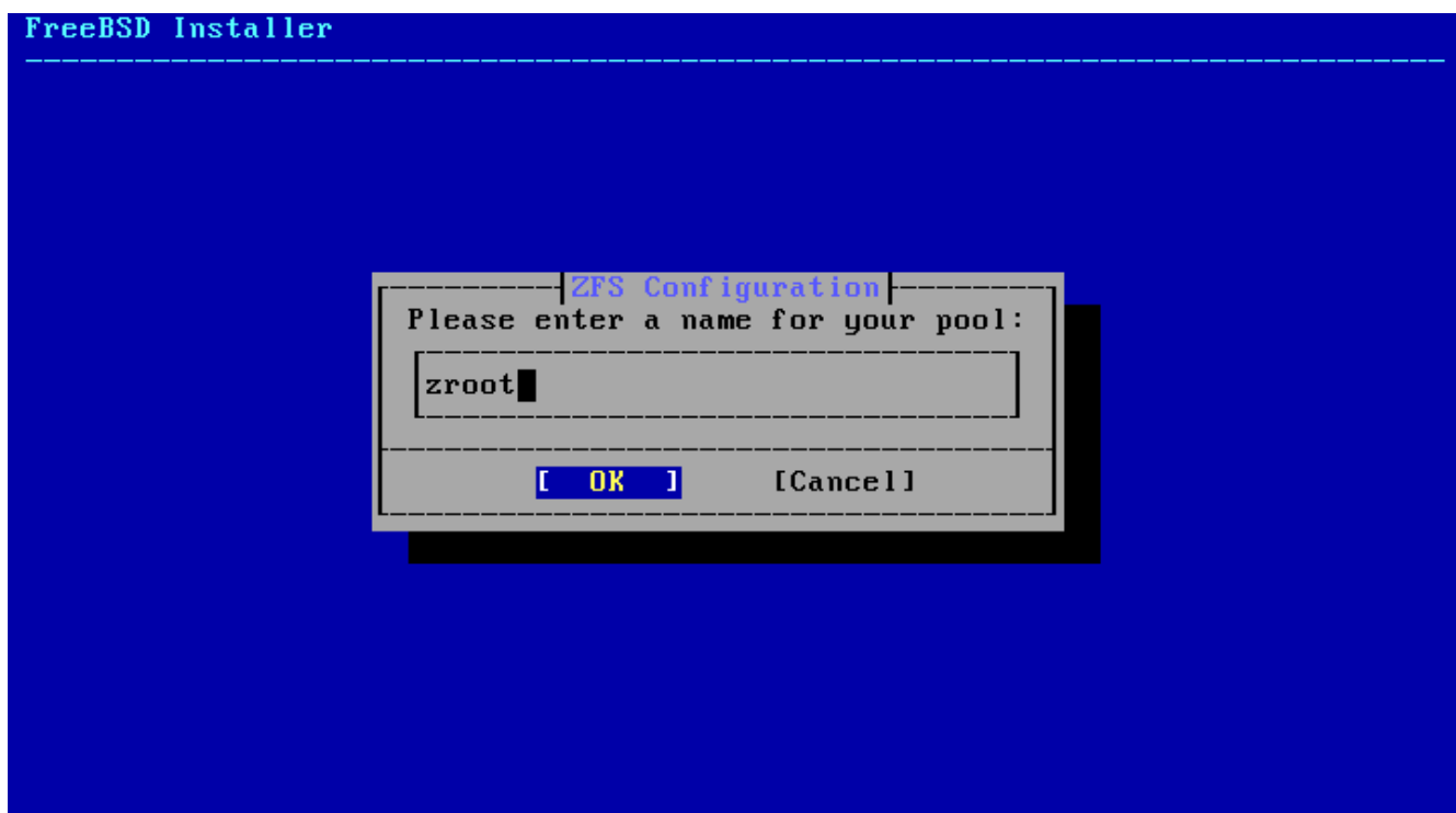
図 26. Pool Name
