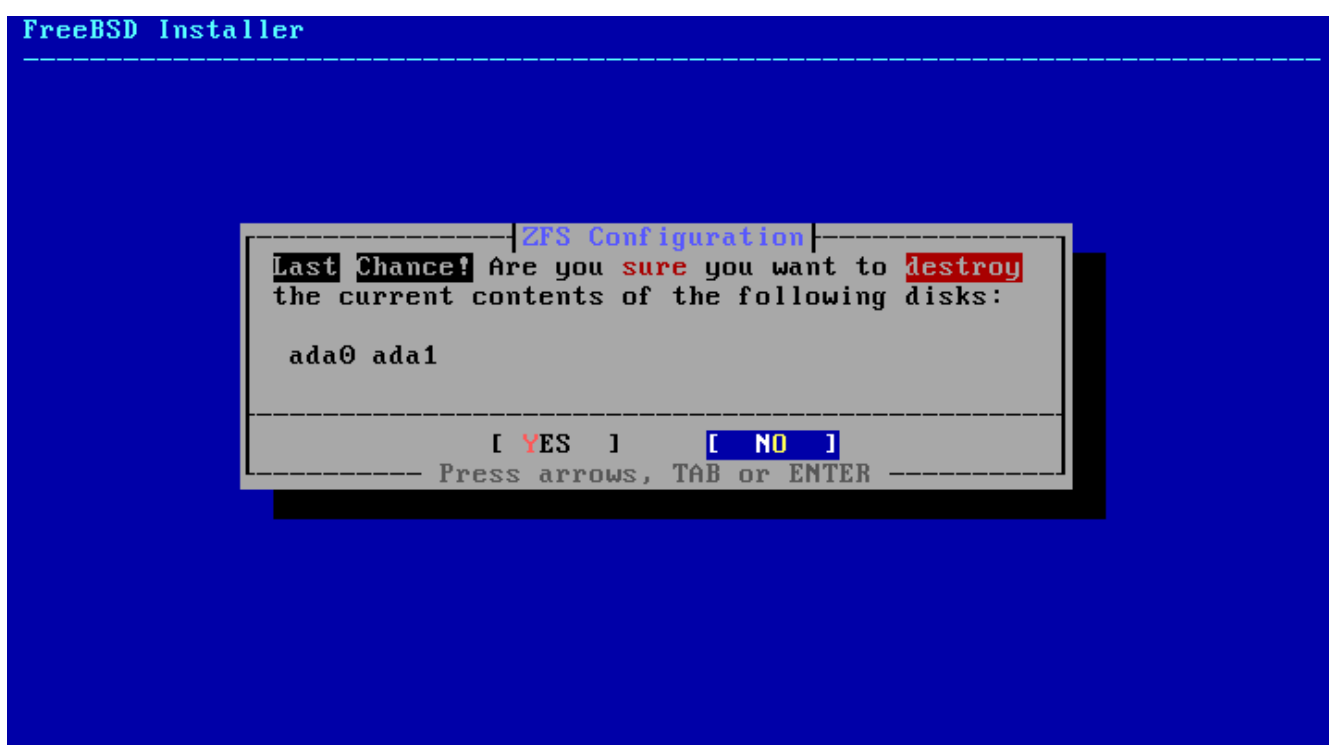
図 28. 最終確認
