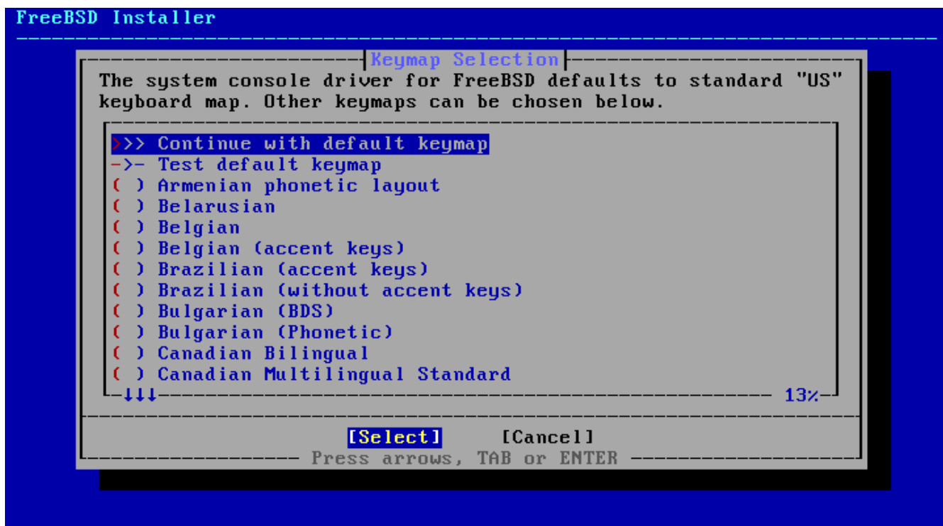
図 5. キーマップ選択メニュー
