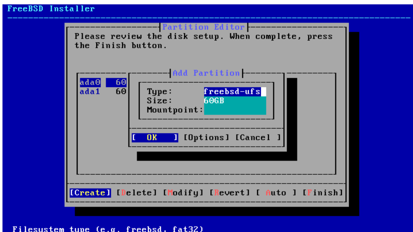
図 19. 手動でパーティションを作成する
