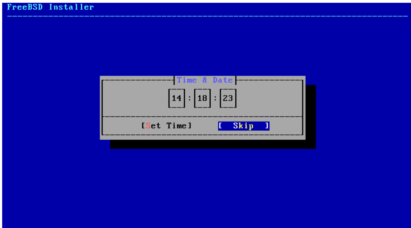
図 52. 時刻の設定
