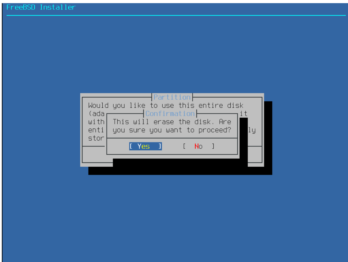
図 13. 確認
