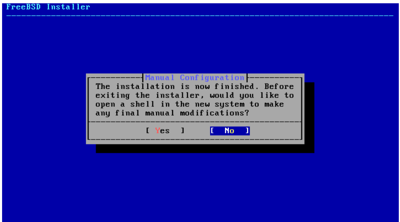
図 58. Manual Configuration
