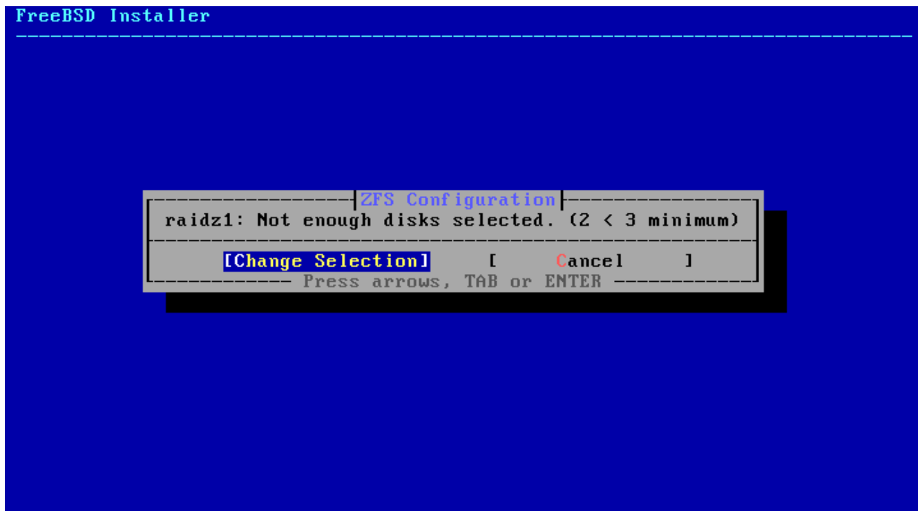
図 23. 無効な選択
