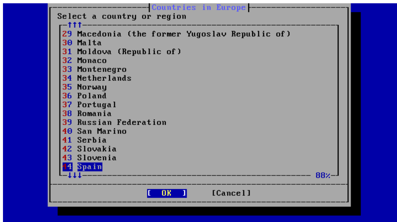
図 48. 国名の選択
