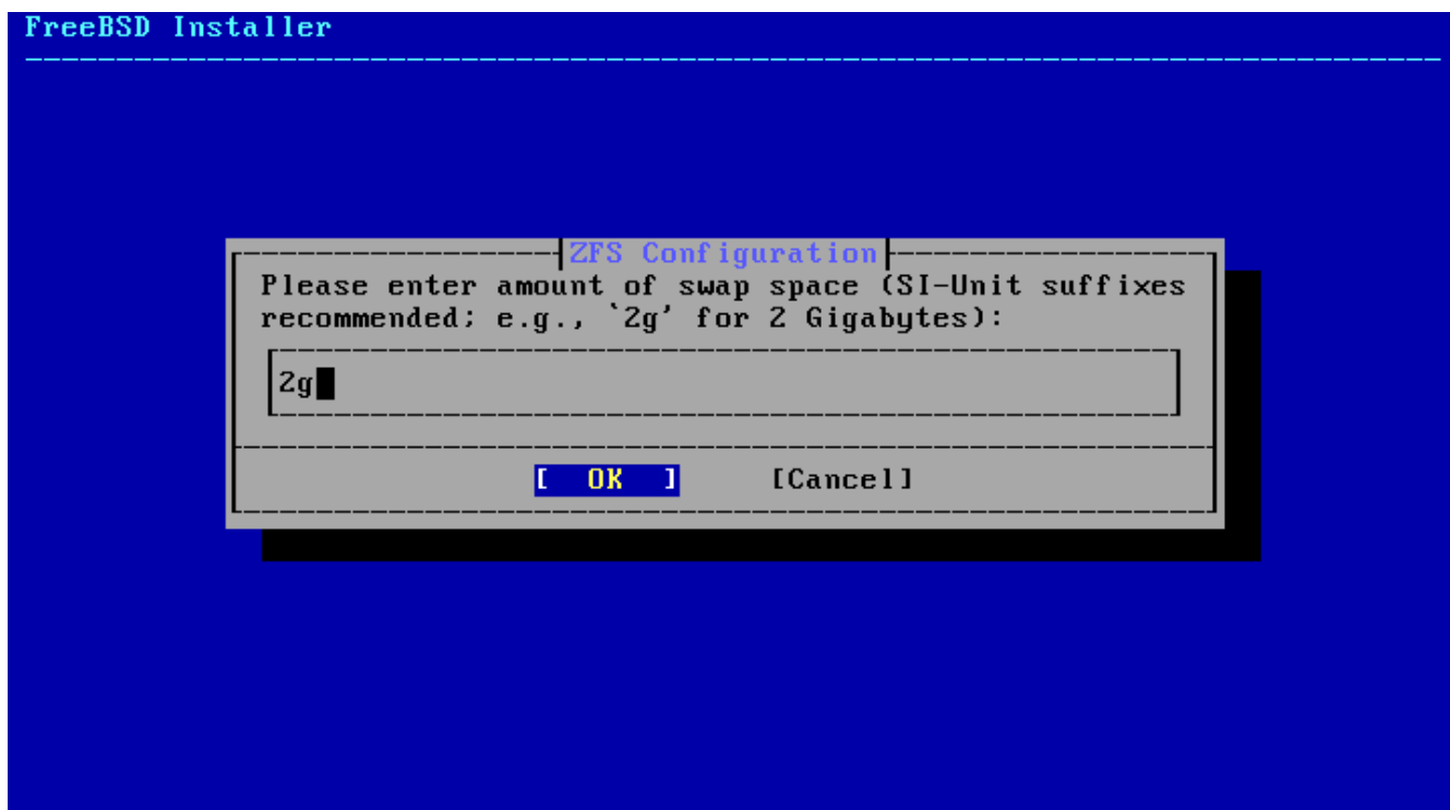
図 27. Swap 容量
